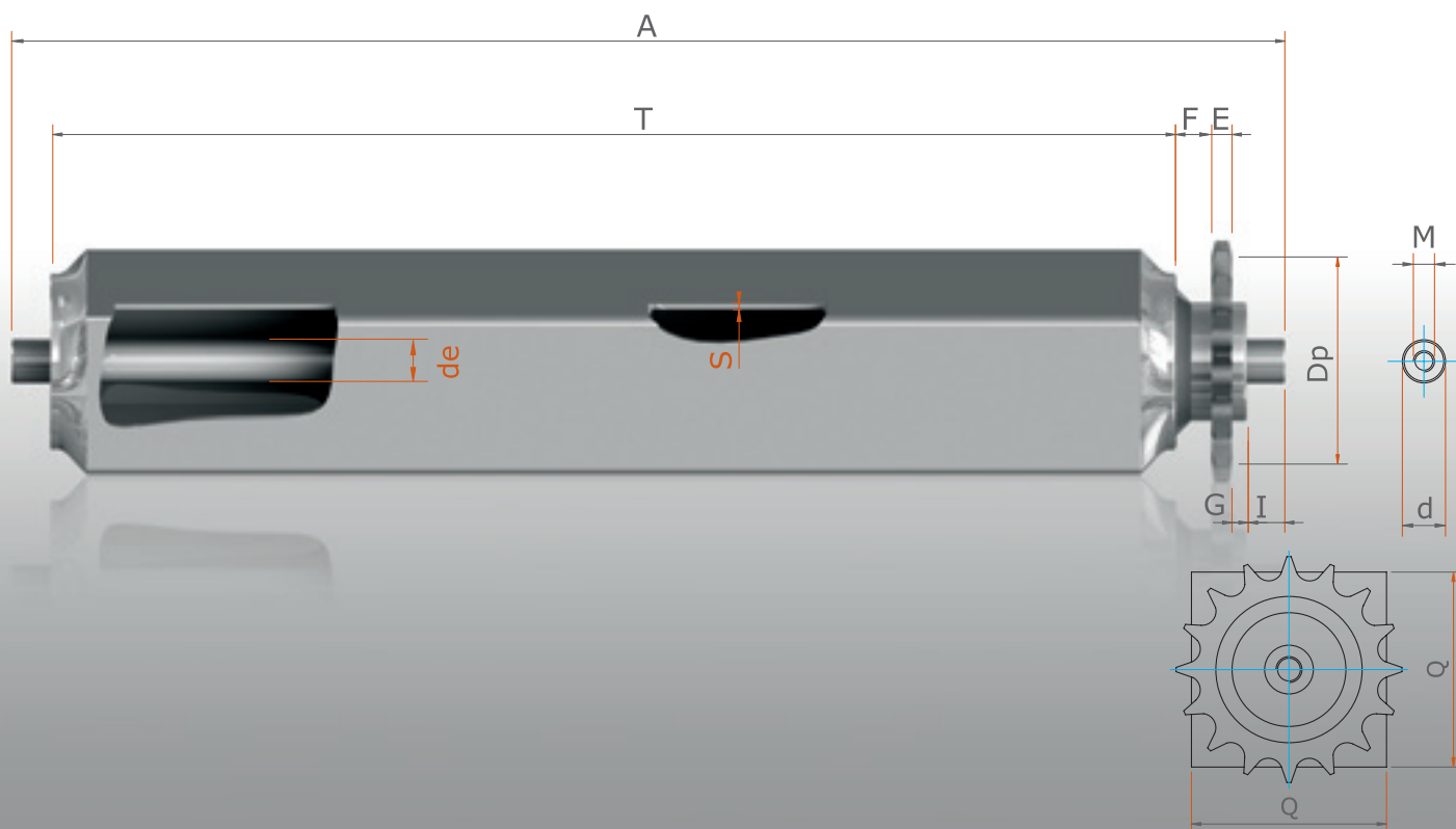
RULLI CON PIGNONE PPSQ - PPSQ PINION SPROCKET ROLLERS
