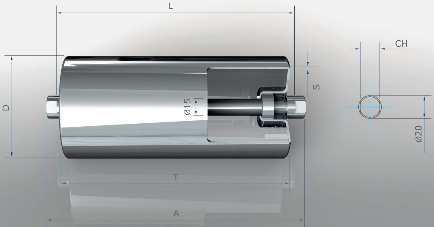
RULLI FOLLI P 200 - P200 IDLER ROLLERS
